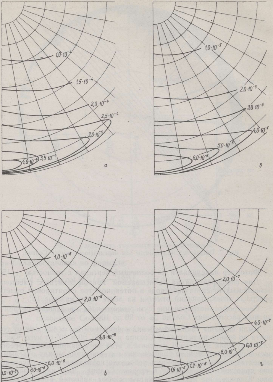
Рис. 8. Изофоты яркостей ( \lambda = 422 мкм) при:
