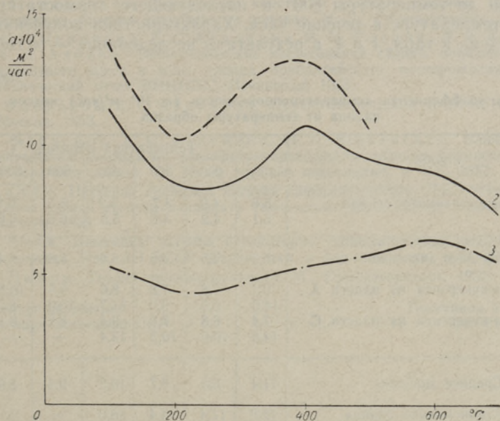
Фиг. 3. Изменение коэффициента теплопроводности с повышением температуры для коксов из: 1 — целика диктионемового сланца; 2 — целика сланца-кукерсита; 3 — прессованного сланца-кукерсита.
