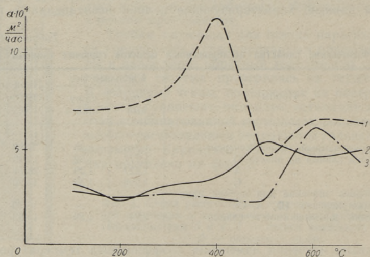
Фиг. 2. Изменение коэффициента температуропроводности с повышением температуры для: 1 — целика диктионемового сланца; 2 — целика сланца-кукерсита; 3 — спрессованного сланца-кукерсита.
