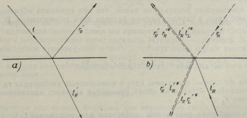
Фиг. 2. К принципу обратимости Стокса.
