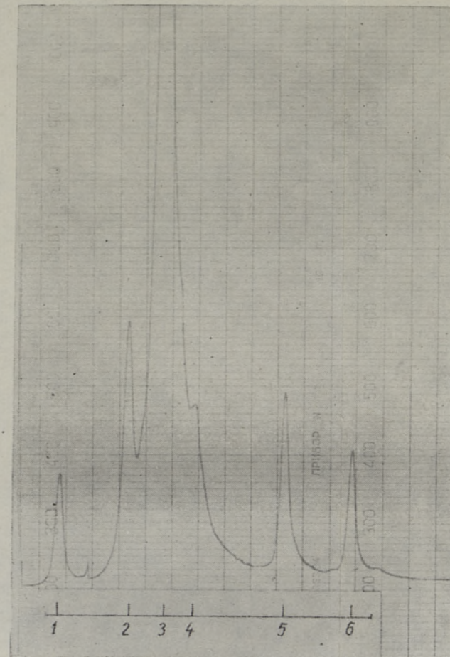
Рис. 5. Спектр ЯМР кислотного остатка этилового эфира коричной кислоты на частоте 40 Мгц.
