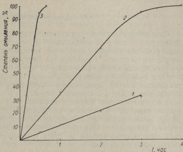
Рис. 2. Зависимость степени омыления сульфохлорида гексахлороктилбициклопентеноктилсульфонилхлорида (глубина сульфохлорирования 52%) от температуры и различных агентов омыления: 1 — 1н. водный раствор NaOH при 20°; 2 — 1н. водный раствор NaOH при 70°; 3 — 1н. этанольный раствор NaOH при 20° (степень сульфохлорирования гексахлороктилбициклопентена 110%). Количество сульфохлорида в каждом опыте составляет 0,02 г-мол; соотношение растворителя (CCl 4 ) к сульфохлориду равно 20. В ходе реакции pH раствора поддерживалась на уровне менее 9.
