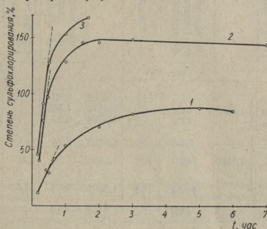
Рис. 1. Зависимость степени сульфохлорирования гексахлоралкилбициклопентенов от времени реакции: 1 — пропилпроизводное; 2 — октилпроизводное; 3 — тетрадецилпроизводное.
