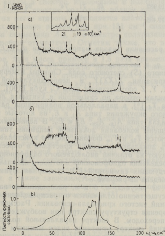
Спектры однофононного рассеяния примесного кристалла \text{KBr}:\text{MnO}_4^- при 5 К в параллельной — Z(XX)Y (а) и перпендикулярной — Z(XZ)Y (б) поляризациях при двух частотах возбуждения — 19932 и 19435 \text{ см}^{-1} (верхние и нижние спектры в а и б соответственно). Спектральная ширина щели — 1,5 \text{ см}^{-1} , регистрация — 10 \text{ с/канал} . а — Теоретическое распределение фоновой плотности в чистом кристалле \text{KBr} . На вставке приведена полоса примесного поглощения примесной молекулы \text{MnO}_4^- в \text{KBr} при 5 К. Стрелками указаны положения частот возбуждения.
