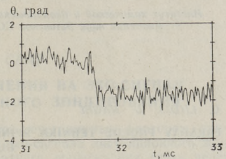
Рис. 5. Участок кривой \theta рис. 4 с временным разрешением 12 мкс.
