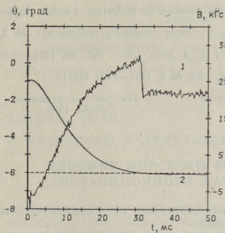
Рис. 4. Поворот Фарадея в СаО при \lambda=335,8 нм и T<0,65 К (1) во время инверсии магнитного поля (2).
