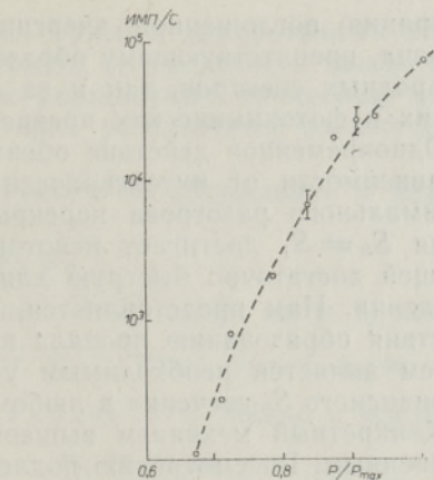
Рис. 2. Резкая (пороговая) зависимость интенсивности S_2 -свечения от относительной мощности возбуждения. P_{\max} \approx 15 мВт (соотв. пиковая интенсивность 0,6 МВт \cdot см ^{-2} ).
