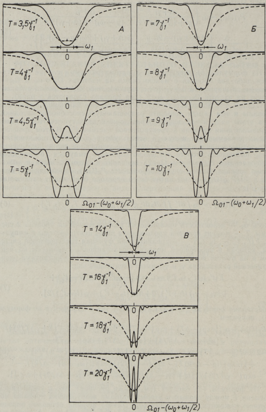
Провалы в ФНР \rho(\Omega_{01}) при двухступенчатом (сплошная линия) и одноступенчатом (штриховая линия) процессах. ( \Delta = 0,99 \gamma_1 ). А — \omega_1 = \gamma_1 ; Б — \omega_1 = 0,5 \gamma_1 ; В — \omega_1 = 0,25 \gamma_1 .
