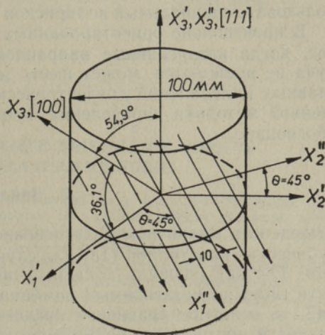
Схема просвечивания цилиндра.
