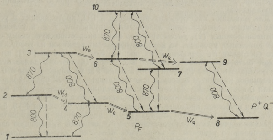
Рис. 1. Схема энергетических уровней РЦ: 1 — основное состояние системы; 2 и 4 — возбужденные уровни P_{800} и P_{870} ; 3 — их совместное возбуждение; 5—7, 10 — основной и возбужденные уровни состояния P_F ; 8 и 9 — основное и возбужденное состояния P^+Q^- . W_e , W_q и W_m — скорости продольной релаксации.
