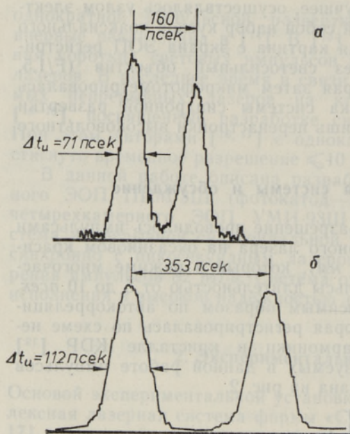
Рис. 3. Микрофотограммы измеренных с помощью ПИМ-3Ш в режиме синхронной развертки импульсов лазера на красителе (а) и Kr^+ -лазера (б). \Delta t_u соответствует измеренной длительности импульсов на полувысоте интенсивности.
