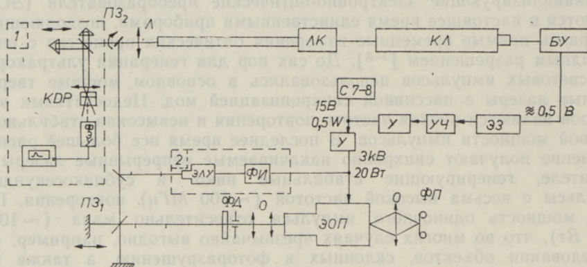
Рис. 1. Схема экспериментальной установки. Обозначения: КЛ — Кг + -лазер, ЛК — лазер на красителе, БУ — блок управления оптикоакустическим модулятором, УЧ — удвоитель частоты, У — усилитель, ЭЗ — узел электрической задержки, Л — линза, О — объектив, ПЗ — полупрозрачное зеркало, Ф — фильтр, Д — диафрагма, ФП — фотоприставка. Отдельно выделены: 1 — автокоррелятор и 2 — система импульсной развертки ЭОП.
