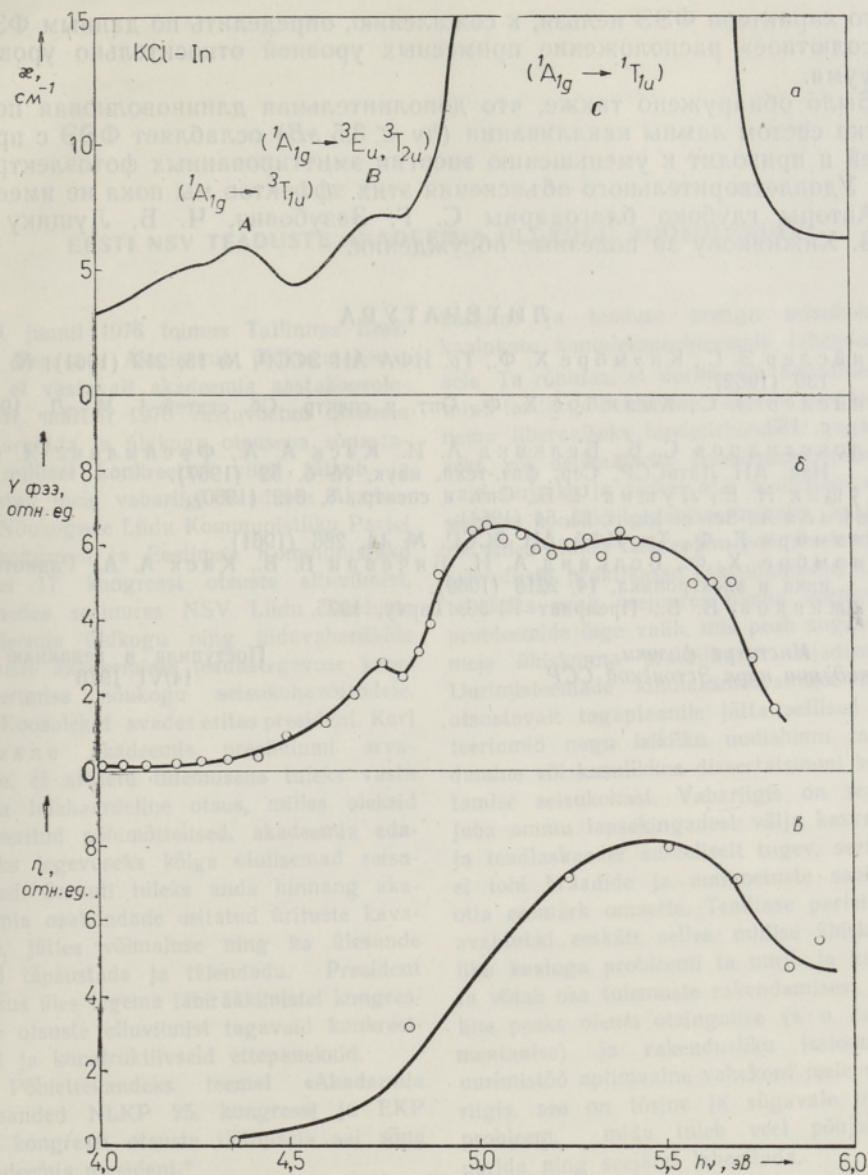
a — Спектр поглощения \text{In}^+ -центров в KCl-In (0,3 мол. % в расплаве), идентификация полос поглощения по данным [4, 5]; b — спектр относительного квантового выхода фотоэлектронной эмиссии с KCl-In; в — спектр создания центров фотостимулированной электронной эмиссии с KCl-In.
