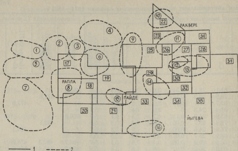
Расположение расчетных площадей. Временно-пространственные группы эксплуатационных (1) и картировочных (2) скважин.
