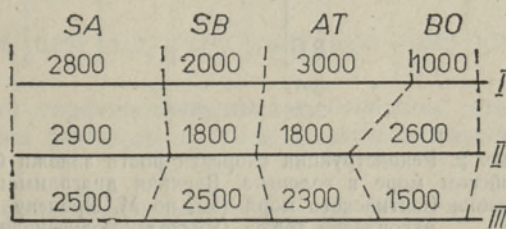
Рис. 1. Продолжительность климатических периодов (годы): I — по местной стратиграфической схеме Эстонской ССР (Каяк и др., 1976), II — по У. Вальку (Valk, 1974), III — по К. Ю. Веберу (1967).
