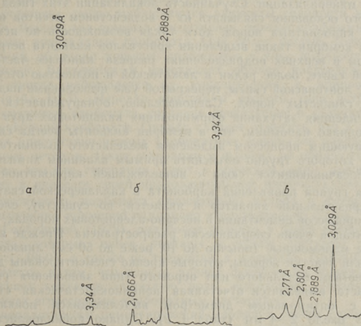
Рис. 1. Дифрактограммы карбонатных минералопоявлений в каллавереской свите. а — жеода в песчанике (Маарду); б — доломитовый цемент песчаника (Маарду); в — пойкилокластический цемент песчаника из западной части Северной Эстонии (скв. Табасалу Ф-294, гл. 126 м).
