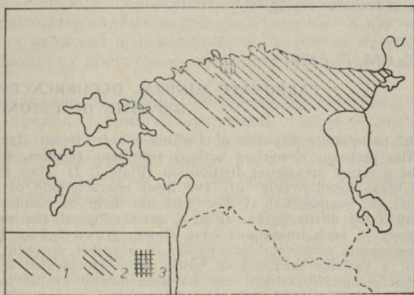
Рис. 3. Предварительное районирование территории Северной Эстонии по типам карбонатпроявлений. 1 — распространение преимущественно кальцитового цемента; 2 — распространение доломитового цемента; 3 — находки жеодово-секрционных образований.
