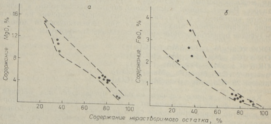
Рис. 2. Зависимость содержания магния (а) и железа (б) в солянокислом растворе от содержания нерастворимого остатка образцов.
