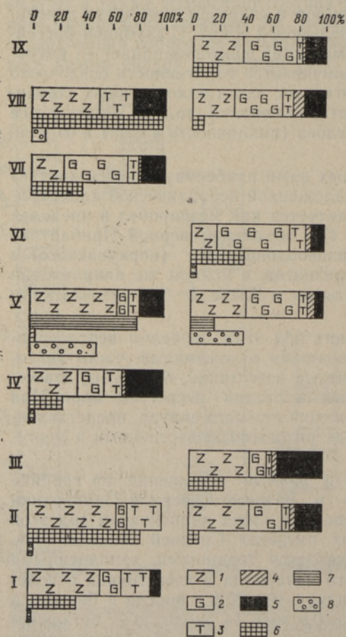
Рис. 2. Содержание основных аутигенных и тяжелых аллотигенных минералов. Разрез скв. Сулуствере: I — поркунский горизонт, гл. 111,0 м; II — граница ордовика и силура гл. 110,3 м, подконтактные (левая сторона) и надконтактные слои (правая сторона); III — юрусский горизонт, гл. 109,7 м; Соомевере: IV — райккюла-ский горизонт, гл. 14,3 м; V — граница адавереского и райккюлаского горизонта, гл. 13,3 м, подконтактные (л. с.) и надконтактные слои (п. с.); VI — адавереский горизонт, гл. 10,0 м; Паатсалу: VII — яагарахуский горизонт, гл. 16,5 м; VIII — поверхность перерыва на гл. 15,0 м, подконтактные (л. с.) и надконтактные (п. с.) слои; IX — яагарахуский горизонт, гл. 9,5 м. 1 — циркон, 2 — гранат, 3 — турмалин, 4 — амфиболы и пироксены, 5 — остальные тяжелые аллотигенные минералы, 6 — пирит, 7 — гематит и гидрогематит, 8 — халцедон.
