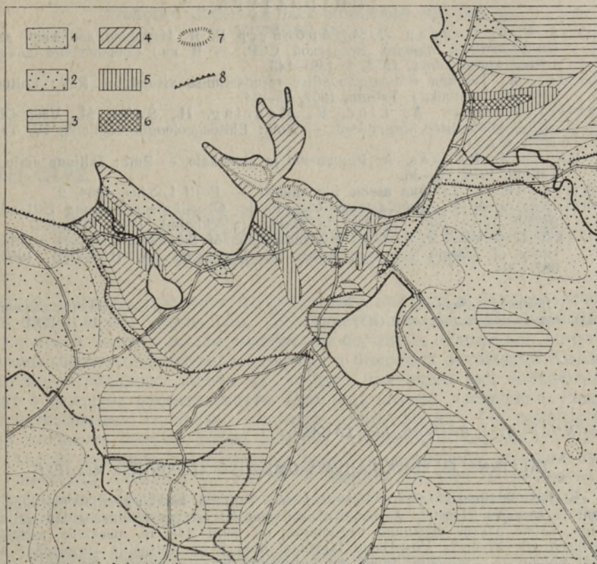
Рис. 3. Схема мощностей четвертичных отложений: 1 — 0—1 м; 2 — 1—5 м; 3 — 5—10 м; 4 — 10—50 м; 5 — 50—100 м; 6 — 100—150 м; 7 — важнейшие возвышения в рельефе коренных пород; 8 — Северо-Эстонский глинт.
