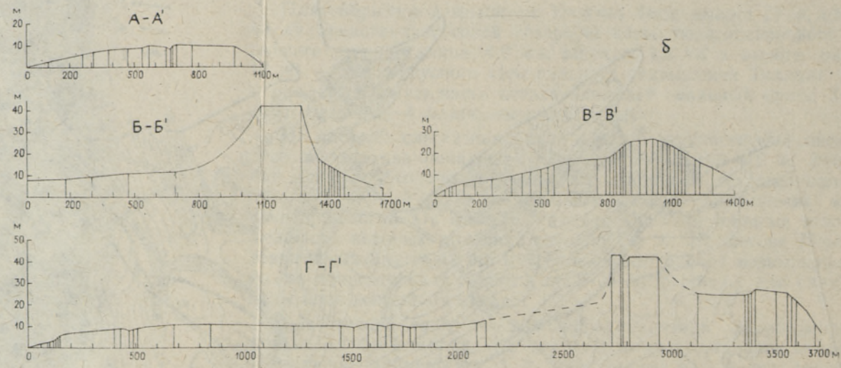
Рис. 2. Морфология Центрального возвышения Таллина (а): 1 — изолинии; 2 — уступы; 3 — абсолютные отметки рельефа поверхности коренных пород, 4 — линии морфологических профилей (б).
