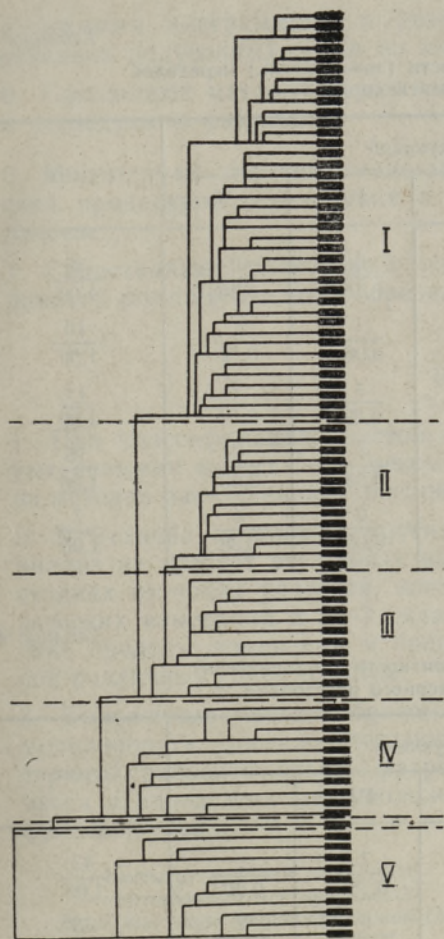
Рис. 1. Классификация разреза V—VII горизонтов месторождения Булла-море по геофизическим параметрам.
