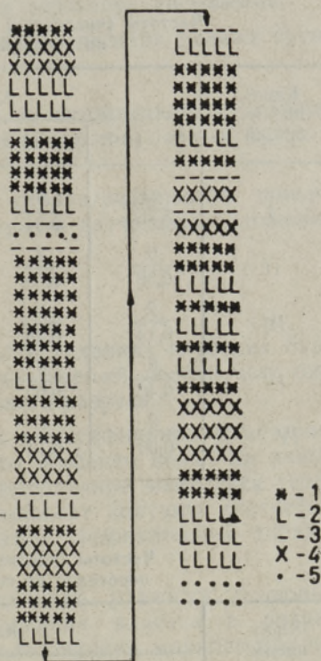
Рис. 2. Моделирование нормального разреза в интервале V—VII горизонтов месторождения Булла-море (скв. 32). 1 — алевритоглинистые пачки; 2 — глины; 3 — коллекторы непродуктивные (глинистые); 4 — коллекторы продуктивные хорошего качества; 5 — коллекторы продуктивные (уплотненные).
