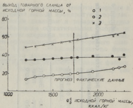
Рис. 4. Зависимость выхода товарных сортов сланца от теплоты сгорания исходной горной массы. 1 — технологический сланец, 2 — энергетический сланец, 3 — технологический и энергетический сланец суммарно.
