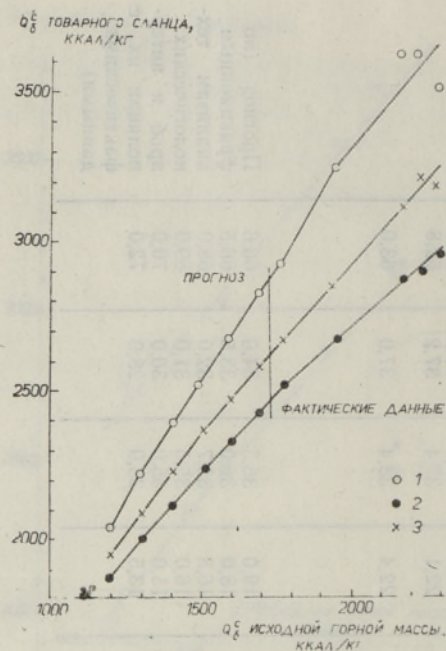
Рис. 3. Зависимость теплоты сгорания товарных сортов сланца от теплоты сгорания исходной горной массы. 1 — технологический сланец, 2 — энергетический сланец, 3 — технологический и энергетический сланец суммарно.
