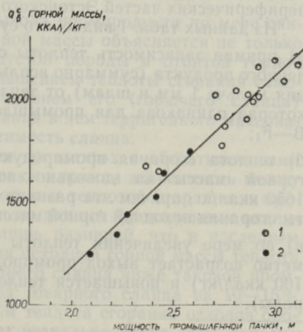
Рис. 1. Корреляция между мощностью и теплотой сгорания горной массы промышленной пачки горючего сланца А—Г. 1 — средние значения пластово-дифференциальных опробований промышленной пачки сланца в горных выработках шахт и разрезов Эстонского месторождения, 2 — средние значения пластово-дифференциальных опробований промышленной пачки сланца по разведочным скважинам на Восточном участке южной части Эстонского месторождения.
