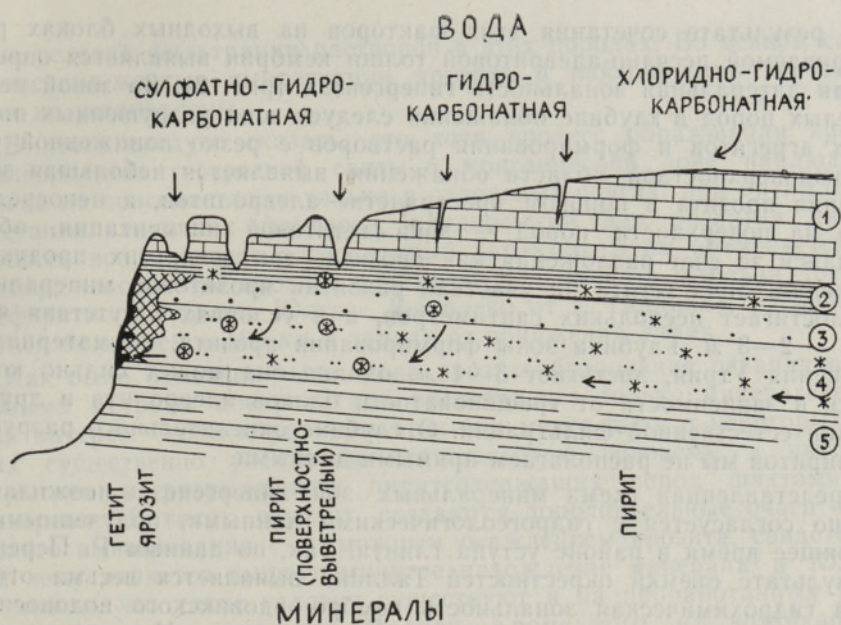
Рис. 2. Принципиальная схема зональности минералообразования и химизма грунтовых вод в районе Северо-Эстонского глинта. 1 — известняк, 2 — граптолитовый (диктиномемовый) сланец, 3 — песчаники пакерортского горизонта ордовика, 4 — алевролиты тискреской свиты кембрия, 5 — глины и алевролиты люкатиской свиты кембрия.
