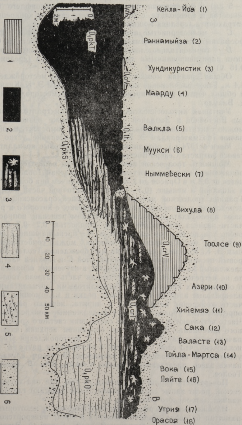
Рис. 1. Разрез верхнетремадокских отложений в обнажениях на глинте. 1 — глины агеритовые зеленовато-серые, 2 — аргиллиты граптолитовые темно-коричневые, 3 — то же с конкрециями антракнита и пирита и прослоями светлых кварцевых агеритов, 4 — агеритовые кварцевые с прослоями граптолитовых аргиллитов, 5 — песчаники кварцевые преимущественно среднезернистые косослонистые с детритом брахиопод, 6 — песчаники кварц-глаукоконитовые слабоцементированные.
