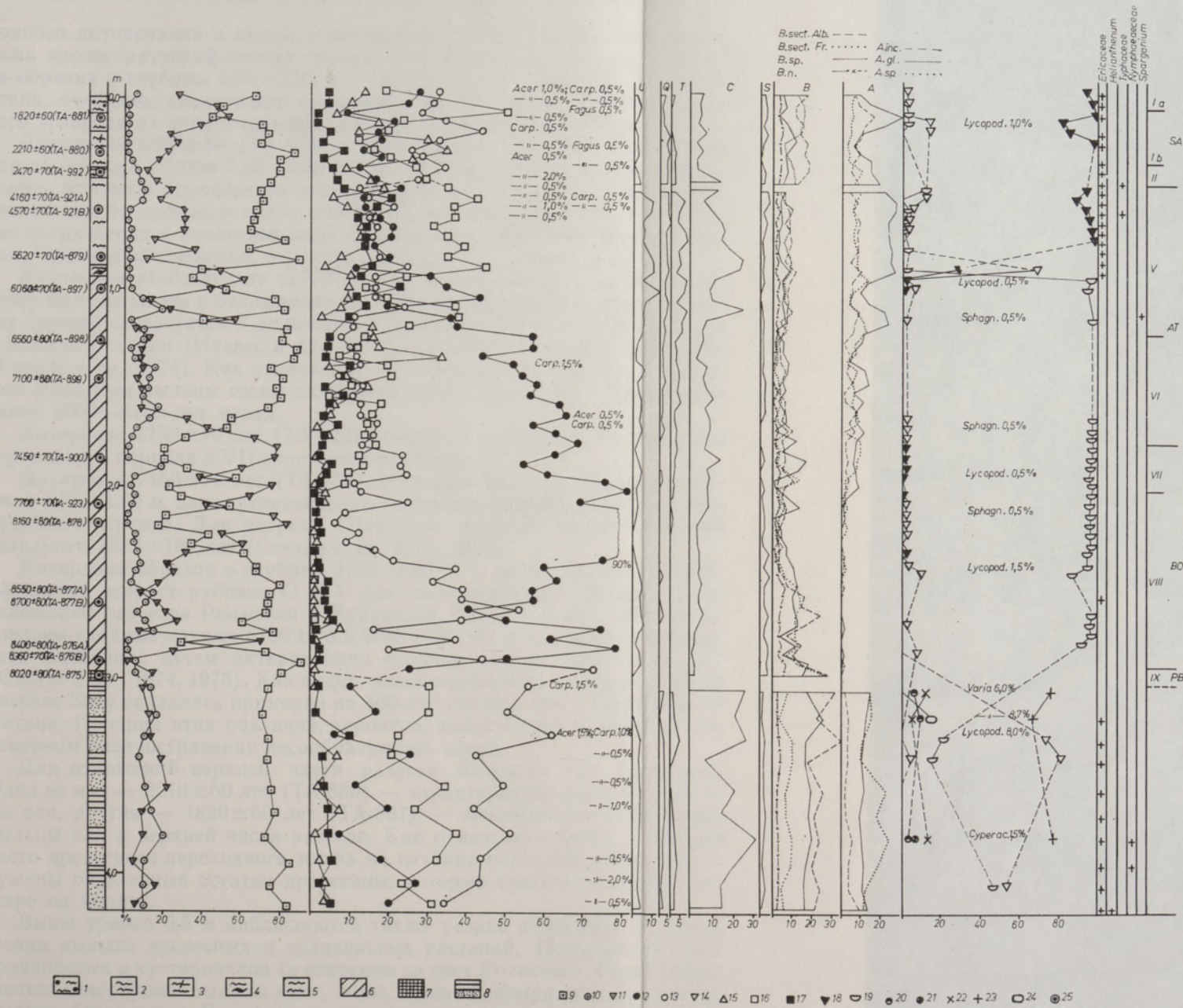
Спорово-пыльцевая диаграмма отложений разреза Зосу. 1 — сосново-сфагновый торф, 2 — комплексный верховой торф, 3 — медуно-торф, 4 — сфагновый переходный торф, 5 — древесный переходный торф, 6 — осоковый торф, 7 — сапрпель, 8 — глина с прослойками песка, 9 — пыльца древесных пород, 10 — споры, 11 — пыльца трав и кустарничков, 12 — сосна, 13 — береза, 14 — ель, 15 — ольха, 16 — широколиственные, 17 — зеленые мхи, 18 — сфагновые мхи, 19 — папоротникообразные, 20 — злаковые, 21 — водные, 22 — маревые, 23 — полыни, 24 — осоковые, 25 — место отбора образца для анализа по 14 C.
