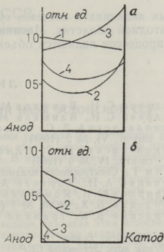
Рис. 3. Распределение интенсивности свечения вдоль канала в различных электролитах: а — \text{NH}_4\text{Cl} ; б — \text{Na}_2\text{S}_2\text{O}_3 ; 1 — \gamma=6,8 \cdot 10^{-3} ом ^{-1} см ^{-1} ; 2 — то же с добавкой орцина (0,2%); 3 — \gamma=2,2 \cdot 10^{-2} ом ^{-1} см ^{-1} ; 4 — то же с добавкой орцина (0,2%); U=22 кв, C=0,32 мкф, l=15 мм.
