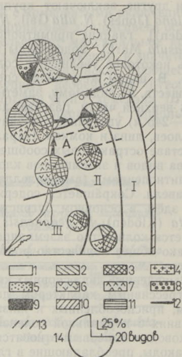
Рис. 4. Сообщества бейрихиид и клоэдениид в даунтонских отложениях Прибалтики.
