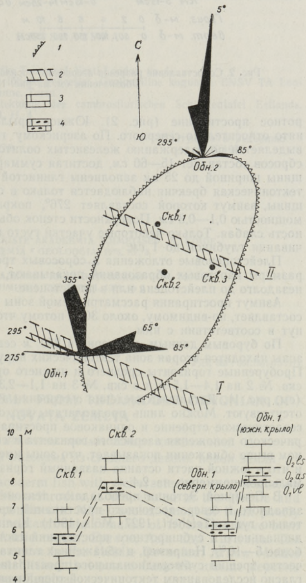
Рис. 1. Тектонические нарушения; роза-диаграммы и геологический разрез останца Тоомпеа: 1 — крутой склон или уступ, 2 — зоны нарушений, 3 — известняк, 4 — оолитовый известняк. Горизонты: O 1 vl — волховский, O 2 as — азерский, O 2 ls — ласнамягский.
