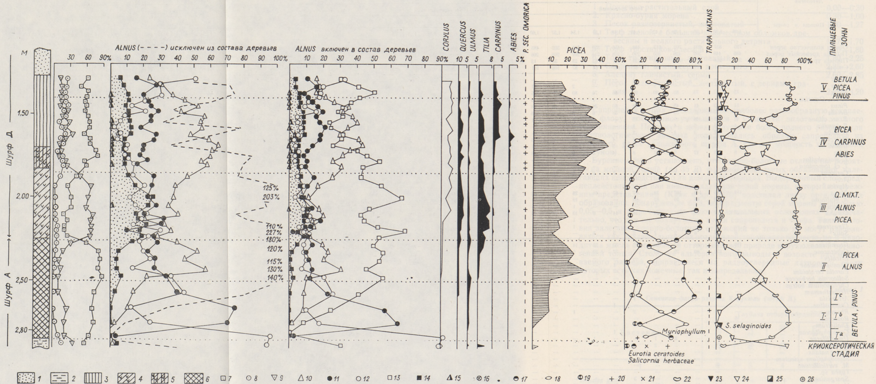
Спорово-пыльцевая диаграмма межледниковых отложений разреза Карукюля: 1 — песок, 2 — алеврит, 3 — древесный торф, 4 — тростниковый торф, 5 — торф переходный, 6 — сапропелит, 7 — пыльца древесных пород, 8 — пыльца трав, 9 — споры, 10 — Picea , 11 — Pinus , 12 — Betula , 13 — Alnus , 14 — Querc. mixt. + Carpinus , 15 — Abies , 16 — Ericales , 17 — Gramineae , 18 — Cyperaceae , 19 — разнотравье ( Varia ), 20 — Artemisia , 21 — Chenopodiaceae , 22 — Polypodiaceae , 23 — Spagnum , 24 — Bryales , 25 — Lycopodium , 26 — Equisetum .
