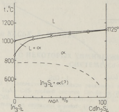
Рис. 3. Фазовая диаграмма разреза \text{In}_3\text{S}_4 — \text{CdIn}_2\text{S}_4 тройной системы Cd—In—S.
