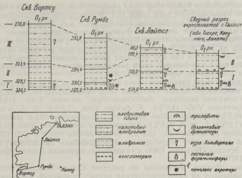
Сопоставление люкатских (I), тискрских (II) и аналогов курземских (III) слоев в разрезах северо-запада Эстонии. (Разрез скв. Виртсу приведен по данным Э. Кала.)
