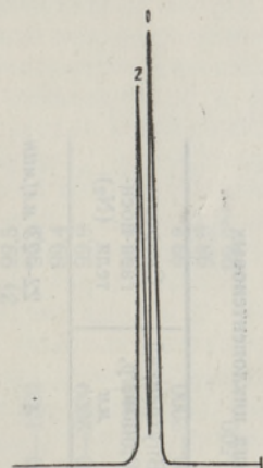
Рис. 2. Хроматограмма геометрических изомеров октена-2. Колонка 1 (см. табл. 1), T 70^{\circ}\text{C} , скорость газа-носителя ( \text{N}_2 ) 60 \text{ мл/мин} . Пики: 1 — октен-2(транс), 2 — октен-2(цис).
