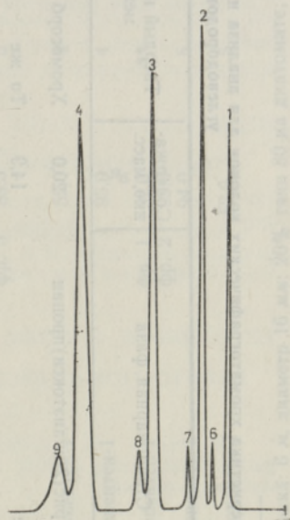
Рис. 3. Хроматограмма смеси 1-алкилциклопентенов. Колонка 1 (см. табл. 1), T 75^{\circ}\text{C} , скорость газа-носителя ( \text{N}_2 ) 55 \text{ мл/мин} . Пики: 1 — 1-этилциклопентен, 2 — 1- n -пропилциклопентен, 3 — 1- n -бутилциклопентен, 4 — 1- n -амилциклопентен, 6—9 — соответствующие алкил-иденциклопентаны.
