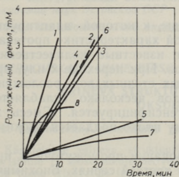
Рис. 1. Кинетика биodeградации фенолов различного строения на иле, адаптированном к резорцину. Нумерация кривых соответствует порядковым номерам в таблице.
