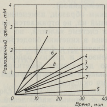
Рис. 2. Кинетика биodeградации фенолов различного строения на иле, адаптированном к промышленным сточным водам. Нумерацию кривых см. в таблице.
