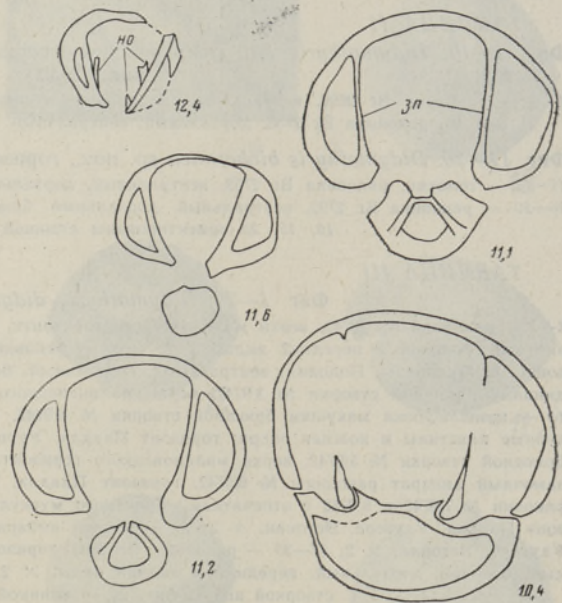
Рис. 3. Последовательные шлифовки примакущечной части раковины Вг 2557 Didymothyris katriensis (поперек смычной поверхности), горизонт Паадла, биогерма Катри (обозначения согласно рис. 2).
