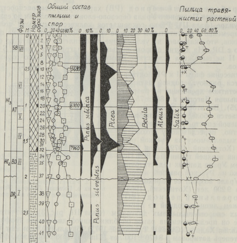
Рис. 3. Спорво-пыльцевая диаграмма разреза бугристого торфяника у оз. Малая Хадата. Условные обозначения те же, что и на рис. 1.
