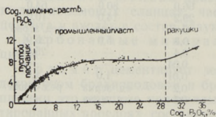
Рис. 1. Зависимость содержания лимонно-растворимого P_2O_5 от содержания P_2O_5 в фосфоритоносных песчаниках.
