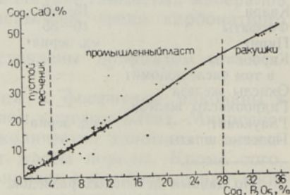
Рис. 2. Зависимость содержания CaO от содержания P_2O_5 в фосфоритоносных песчаниках.
