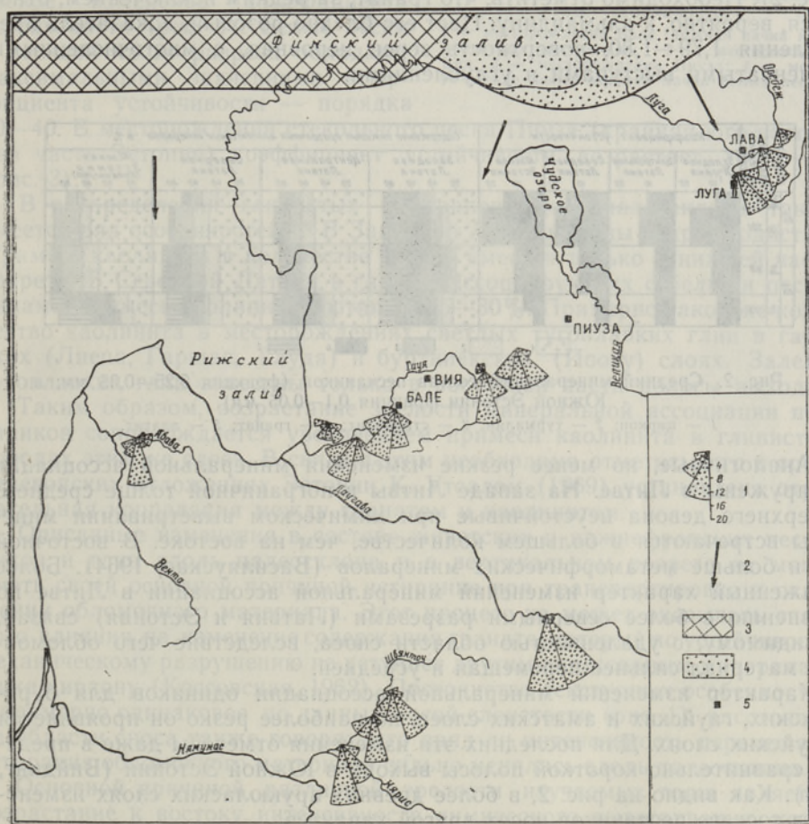
Рис. 1. Направление сноса обломочного материала в гаульское время по данным изучения косої слоистости.
