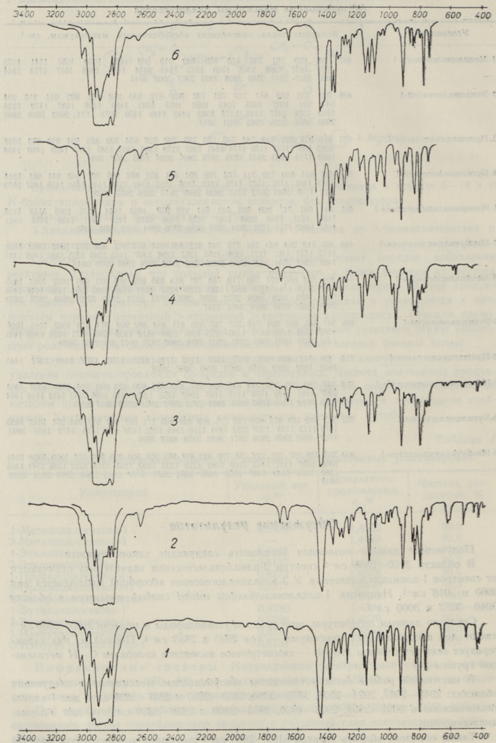
Рис. 1. Инфракрасные спектры 1-алкилциклогексенов:
