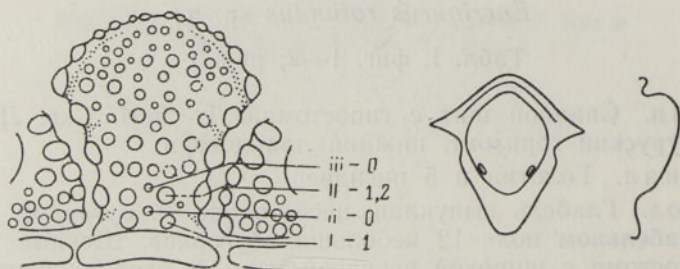
Рис. 1. Расположение бугорков на глабели и строение гипостомы Encrinurus rotundus sp. n. Индексация бугорков по системе Р. Триппа (Tripp, 1957).
