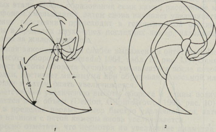
Рис. 2. Схемы строения фрагмокона эмбриональных раковин: 1 — Nautilus pompilius L. ( \times 3,1 ), рисунок сделан по начальной части раковины экз. № Со 11; d — диаметр эмбрионального фрагмокона, pr — длина умбонального отверстия, nl — его ширина, k — высота оборота, sk — расстояние сифона от вентральной стороны раковины, p — длина воздушной камеры. 2 — Nautilus macromphalus Sow. ( \times 2,9 ), рисунок сделан по начальной части раковины экз. № Со 25.
