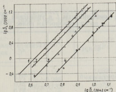
Рис. 2. Зависимость \lg \bar{D}_L при 3350 \text{ см}^{-1} от \lg \bar{D}_1 при 3642 \text{ см}^{-1} для n -пропилового спирта. 1 — 20,5^\circ , 2 — 25^\circ , 3 — 35^\circ , 4 — 50^\circ .
