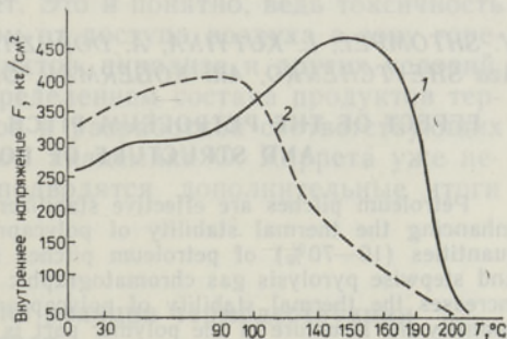
Рис. 2. Изменение внутренних напряжений в поликапроамидной нити (1) и в нити из композиции поликапроамид—пек (2).
