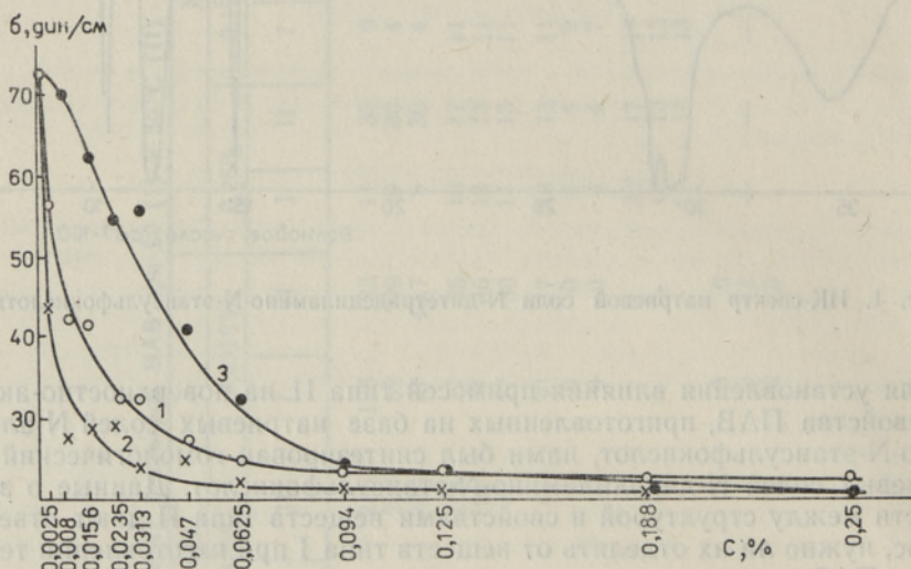
Рис. 2. Изотермы поверхностного натяжения ( \sigma ) водных растворов натриевых солей N-диоктиламино- (1), N-дидециламино- (2) и N-дидодециламино-N-этансульфокислот (3).
