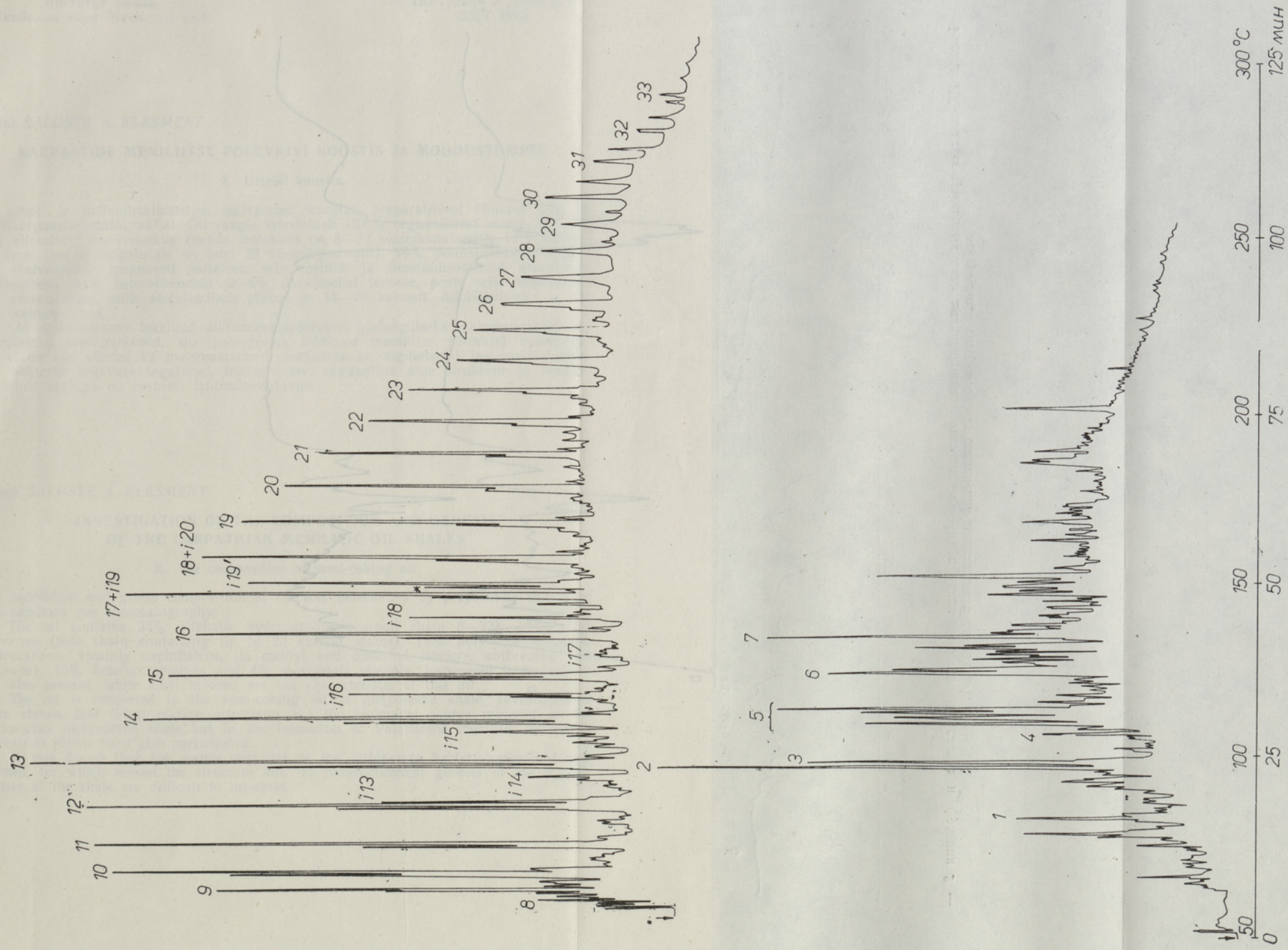
Рис. 1. Хроматограммы фракций неароматических углеводородов (а) и полициклических ароматических углеводородов (б). Колонка: 15 м (Ø 0,25 мм) дексил 300, повышение температуры в колонке — 2 град/мин. Цифры 8—32 указывают на число атомов углерода в молекуле n -алкана и n -алкена; цифры 13—120 — число атомов углерода в молекуле изопреноидного углеводорода; 119' — пристен-1; * — изомер пристена; 1 — нафталин; 2 — 2-метилнафталин; 3 — 1-метилнафталин; 4 — дифенил; 5 — диметилнафталины; 6 — аценафтен; 7 — флуорен.
