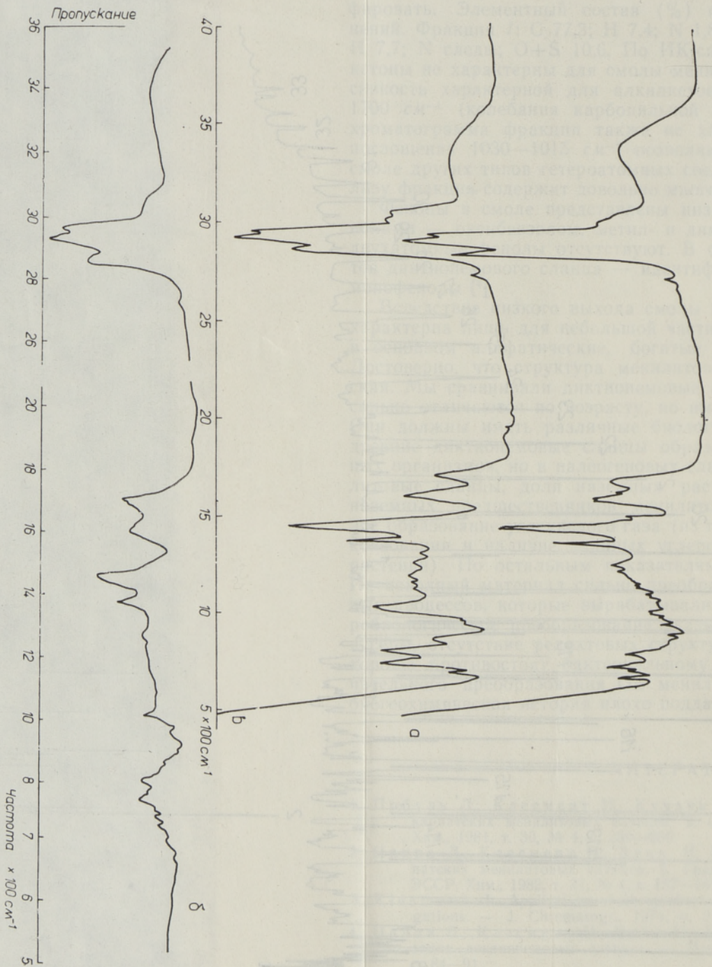
Рис. 2. ИК-спектры суммарных смол полужокования менлитового (а) и диэтионемового (б) сланца и фракции 2 — нейтральных гетероатомных соединений менлитового сланца (в).
