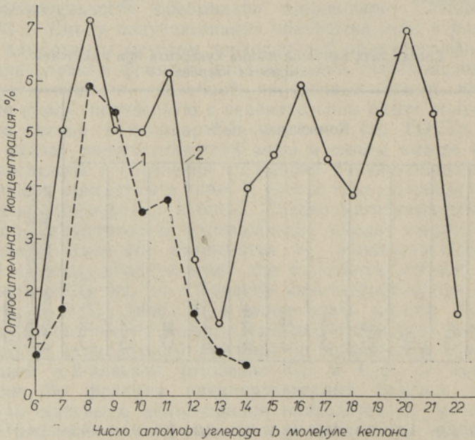
Рис. 2. Распределение по длине цепи метил- n -алкилкетонов (1) и симметричных или близких к ним n -алканов (2) в смоле высокоскоростного полукоксования кукурсита (% их суммарного содержания).
