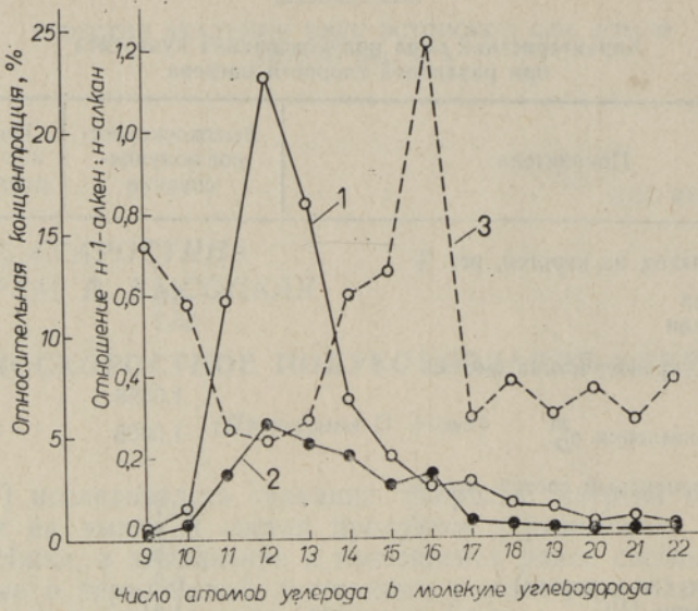
Рис. 1. Распределение по длине цепи n -алканов (1) и n -1-алкенов (2) в смоле высокоскоростного полукоксования кукурсита (% их суммарного содержания) и зависимость величины отношения n -1-алкены: n -алканы от числа атомов углерода в молекуле углеводорода (3).
