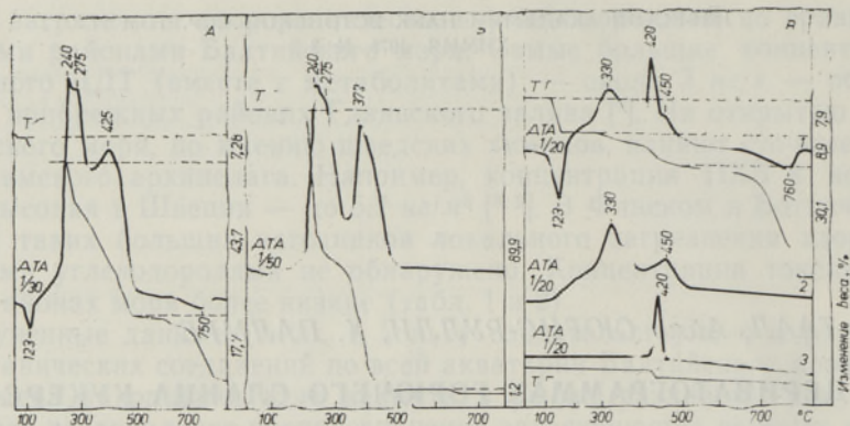
Дериватограммы: А — кукурсита; Б — флотационного концентрата; В — флотационного остатка (1); Al_2O_3 , содержащего 6,7% флотационного концентрата (2); Al_2O_3 , содержащего 6% пирита (3).
