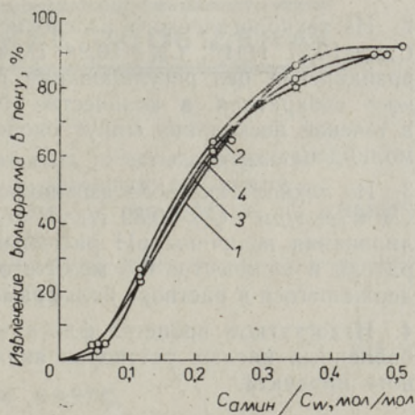
Рис. 2. Флотуемость вольфрама в зависимости от количества прибавляемого гидрохлорида додециламина из технологических растворов, разбавленных 1:9 (кривая 1), 1:4 (2), 1:1 (3), и из неразбавленного раствора (4).
