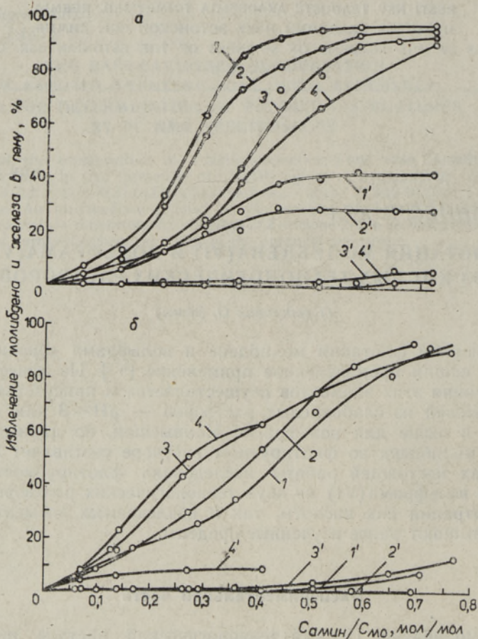
Рис. 1. Флотированность молибдена (кривые 1—4) и железа (кривые 1'—4') в зависимости от количества добавляемого гидрохлорида додециламина: а — из технологического раствора, разбавленного 1:9, при рН 2,2 (кривые 1, 1'), 1,7 (2, 2'), 1,3 (3, 3') и 0,9 (4, 4'); б — из технологических растворов, разбавленных 1:9 (кривые 1, 1'), 1:4 (2, 2'), 1:1 (3, 3'), и из неразбавленного раствора (4, 4') без регулирования рН.
