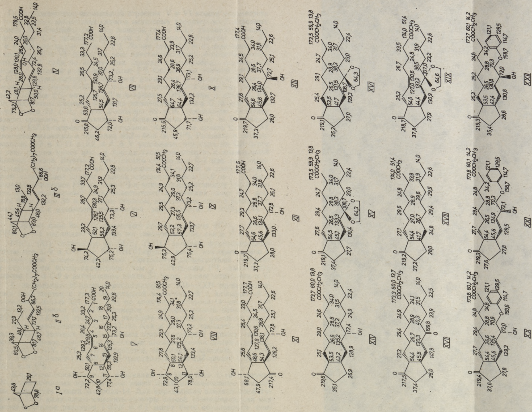
Рис. 1. Химические сдвиги ядер 13 C простагнонов. I — 2,3-диоксациклогло[2,2,1]гептан; II — 5-экто (3-гидроперокси-10-метоксикарбонил-E-2-деннил)-6-экто-этил-2,3-диоксациклогло[2,2,1]гептан; III — 5-эндо (3-гидроперокси-10-метоксикарбонил-E-2-деннил)-6-эндо-этил-2,3-диоксациклогло[2,2,1]гептан; IV — PGH 2 ; V — PGF 2a ; VI — PGF 2β ; VII — PGE 2 ; VIII — PGF 1α ; IX — PGF 1β ; X — PGE 1 ; XI — PGD 2 ; XII — 11-дезоксипGE 1 (15S(α)OH); XIII — 11-дезоксипGE 1 (15R(β)OH); XIV — этиловый эфир-8-изо-11-дезоксипGE 1 ; XV — этиловый эфир-15-этилендиоксипGE 1 ; XVI — этиловый эфир-15-этилендиоксип-9-оксо-8-изо-13E-простеновой кислоты; XVII — этиловый эфир-9,15-диоксо-13E-простеновой кислоты; XVIII — метиловый эфир-9-оксо-простаеновой кислоты; XIX — метиловый эфир-15-этилендиоксип-9-оксо-Z5,13E-простаеновой кислоты; XX — диэтиловый эфир-16-фенокси-17,18,19,20-тетранор-11-дезоксипростагландина E 1 (15S(α)OH); XXI — диэтиловый эфир-16-фенокси-17,18,19,20-тетранор-8-изо-11-дезоксипростагландина E 1 (15R(β)OH); XXII — диэтиловый эфир-16-фенокси-17,18,19,20-тетранор-8-изо-11-дезоксипростагландина E 1 , а данные из [7, 12]; б — химические сдвиги (без отнесения) приведены в [6, 11].
