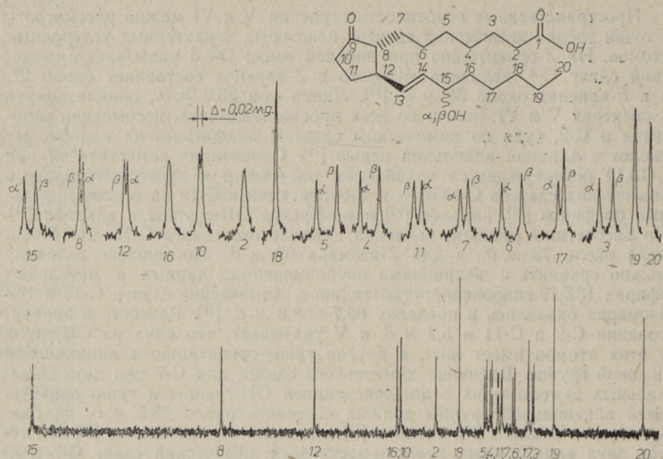
Рис. 2. Спектр ядер насыщенных атомов углерода смеси изомеров 15 \alpha (S)- и 15 \beta (R)-11-дезоксипГЕ 1 .
