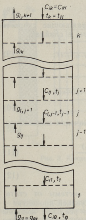
Рис. 1. Разделение реактора на слайды.
