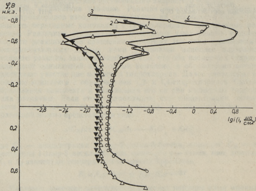
Рис. 1. Анодные поляризационные кривые углеродистой стали в 25%-ном растворе моноэтанолamina (МЭА): 1, 2 — 0,19 моль CO_2 /моль МЭА при 20 °С; 3, 4 — 0,415 моль CO_2 /моль МЭА, 90 °С; 2, 3 — статические условия; 1, 4 — динамические условия.
