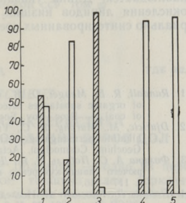
Рис. 4. Соотношение моно- и \alpha\omega -дикарбоксильных кислот в битумоидах балхашита (1, 2, 3) и в продуктах окисления (4, 5). 1 и 4 — черный, 2 и 5 — бурый, 3 — рассеянный балхашит. Заштрихованные колонки соответствуют монокарбоновым кислотам, незаштрихованные \alpha\omega -дикарбоксильным.
