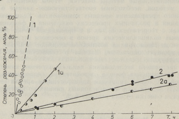
Рис. 1. Кинетика окисления пирокатехина 3 \cdot 10^{-4} моль/л (1) и бенз(а)пирена 5 \cdot 10^{-4} моль/л (2) отдельно и в смеси (а).
